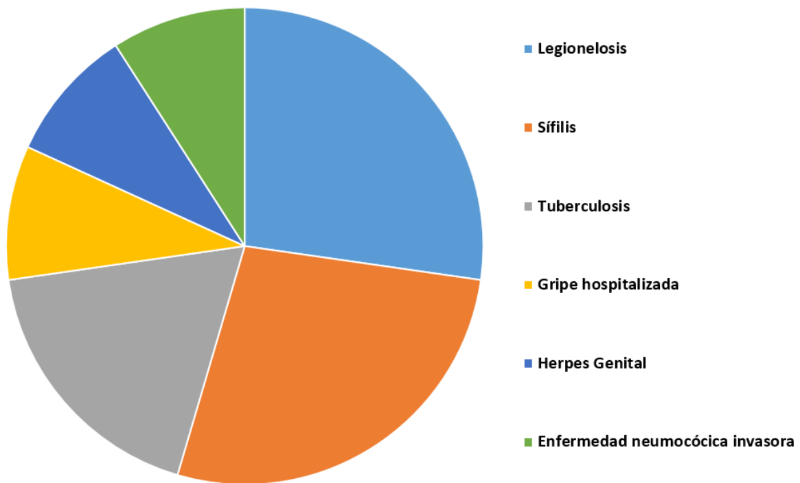
Fig. 23 -. Representación gráfica de EDOs
